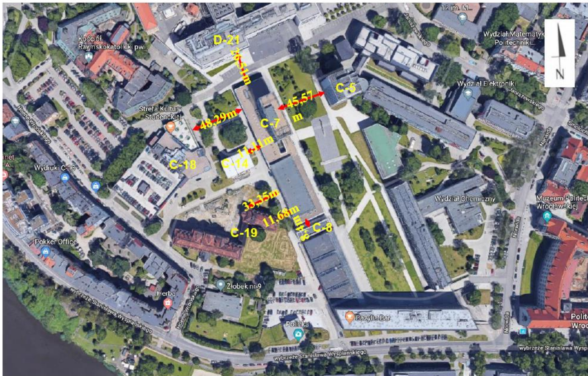
ODLEGŁOŚĆ BUD. C-7 POLITECHNIKI WROCLAWSKIEJ OD OBIEKTÓW SĄSIEDNICH
