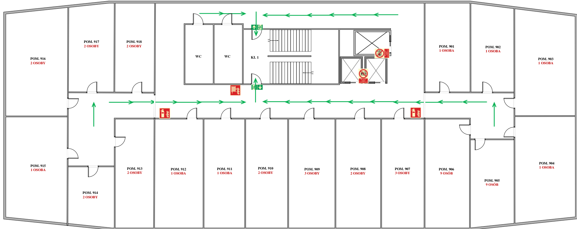
Rozmieszczenie urządzeń przeciwpożarowych oraz kierunków ewakuacji W BUDYNKU C-7 POLITECHNIKI WROCŁAWSKIEJ IX PIĘTRO CZ. A/B
