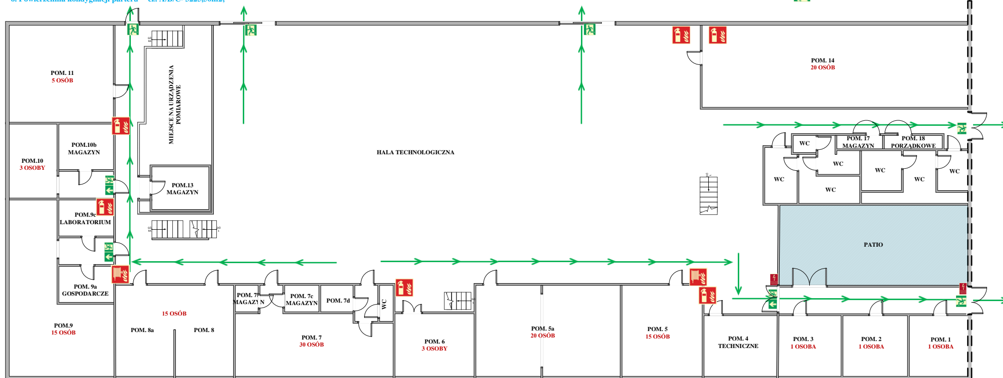
Rozmieszczenie urządzeń przeciwpożarowych oraz kierunków ewakuacji W BUDYNKU C-7 POLITECHNIKI WROCŁAWSKIEJ PARTER CZ. C
