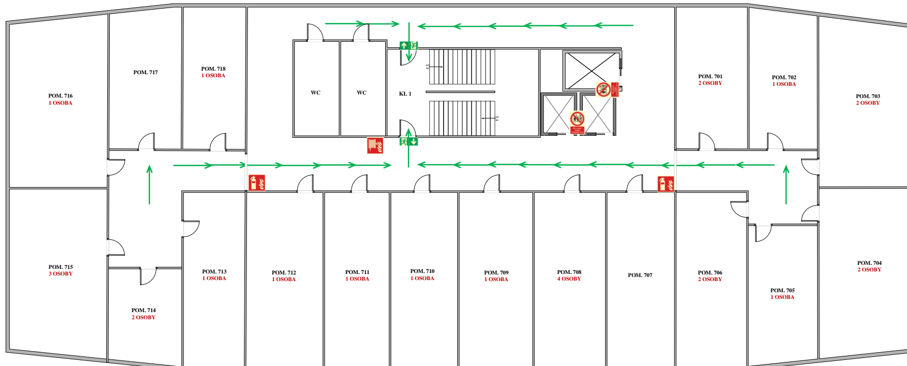
Rozmieszczenie urządzeń przeciwpożarowych oraz kierunków ewakuacji W BUDYNKU C-7 POLITECHNIKI WROCŁAWSKIEJ VII PIĘTRO CZ. A/B
