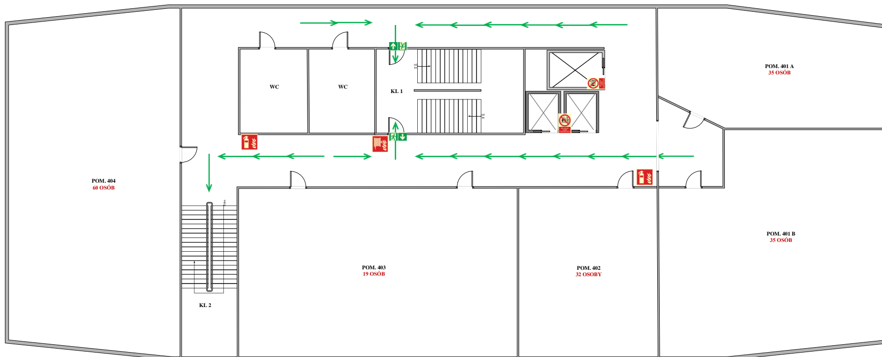
Rozmieszczenie urządzeń przeciwpożarowych oraz kierunków ewakuacji W BUDYNKU C-7 POLITECHNIKI WROCŁAWSKIEJ IV PIĘTRO CZ. A/B
