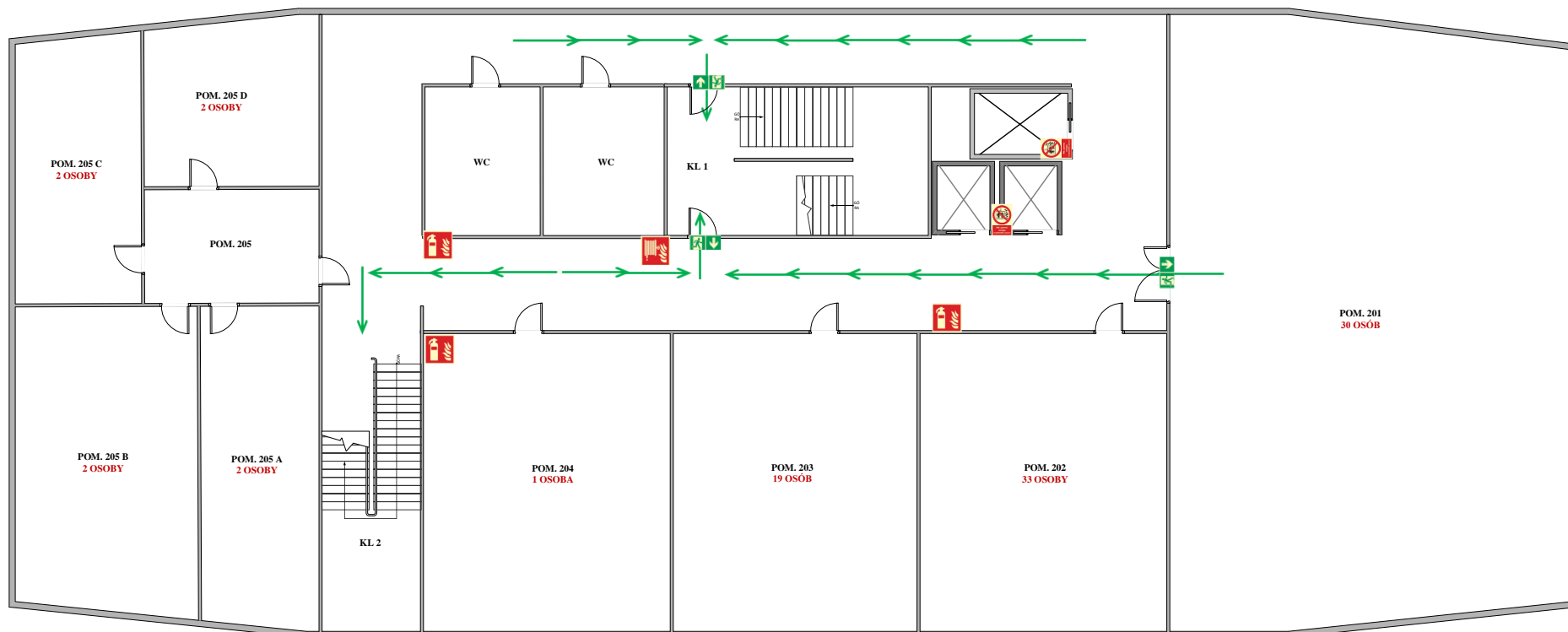
Rozmieszczenie urządzeń przeciwpożarowych oraz kierunków ewakuacji W BUDYNKU C-7 POLITECHNIKI WROCŁAWSKIEJ II PIĘTRO CZ. A/B
