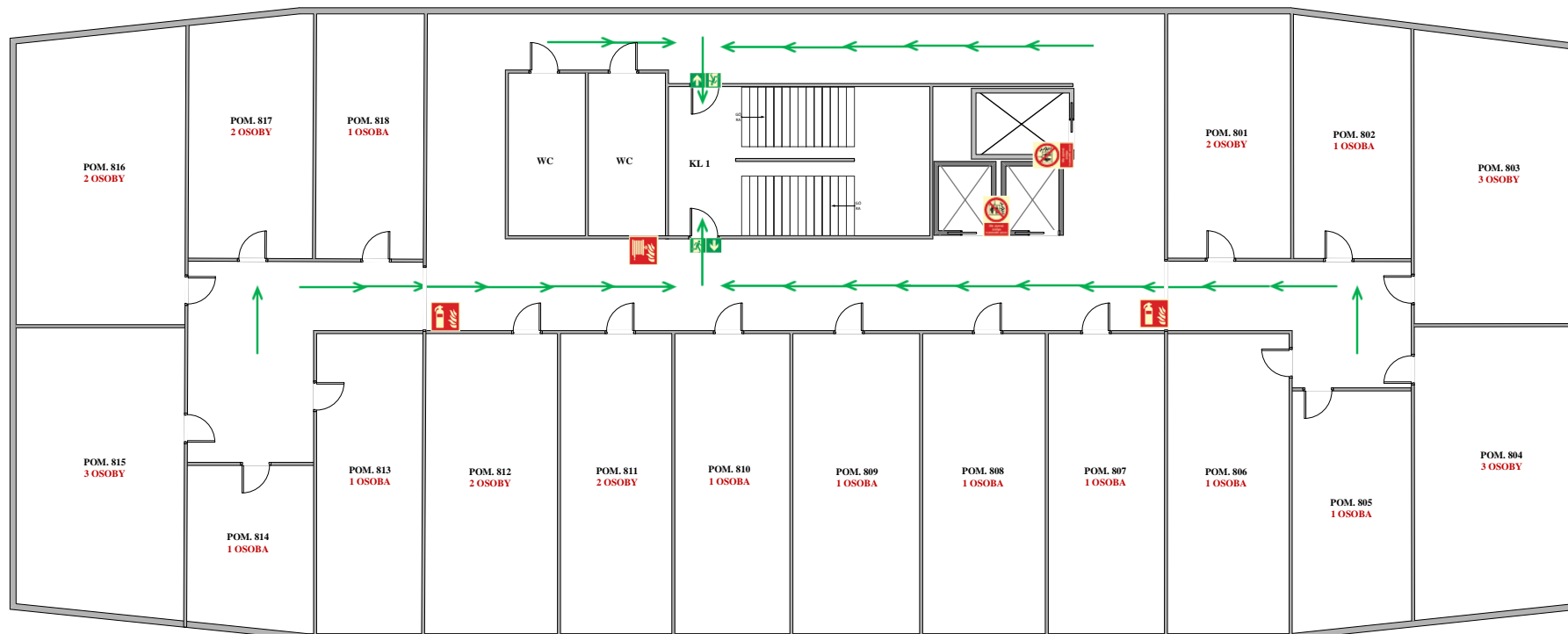
Rozmieszczenie urządzeń przeciwpożarowych oraz kierunków ewakuacji W BUDYNKU C-7 POLITECHNIKI WROCŁAWSKIEJ VIII PIĘTRO CZ. A/B
