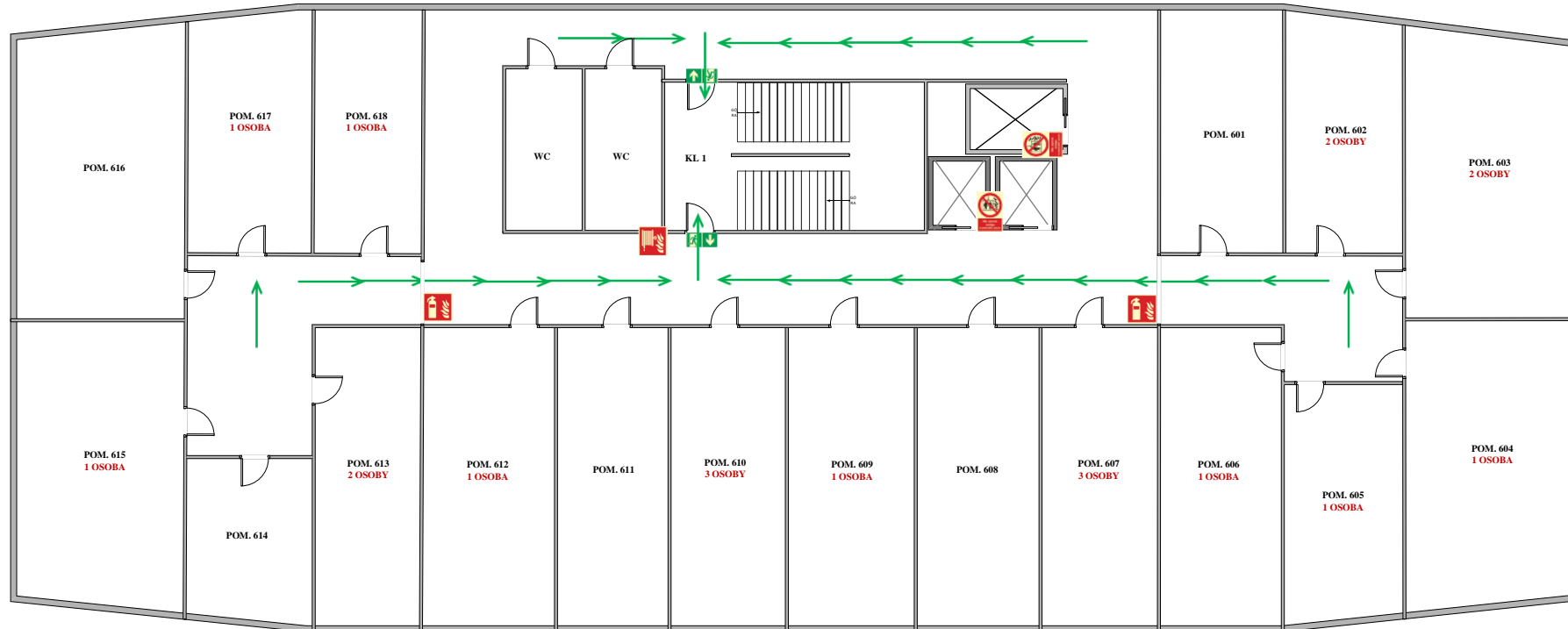
Rozmieszczenie urządzeń przeciwpożarowych oraz kierunków ewakuacji W BUDYNKU C-7 POLITECHNIKI WROCŁAWSKIEJ VI PIĘTRO CZ. A/B
