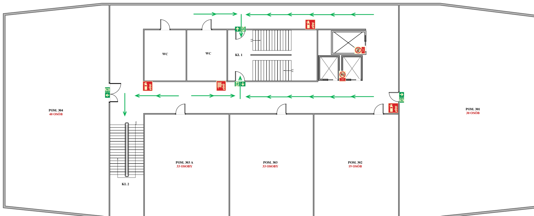
Rozmieszczenie urządzeń przeciwpożarowych oraz kierunków ewakuacji W BUDYNKU C-7 POLITECHNIKI WROCŁAWSKIEJ III PIĘTRO CZ. A/B
