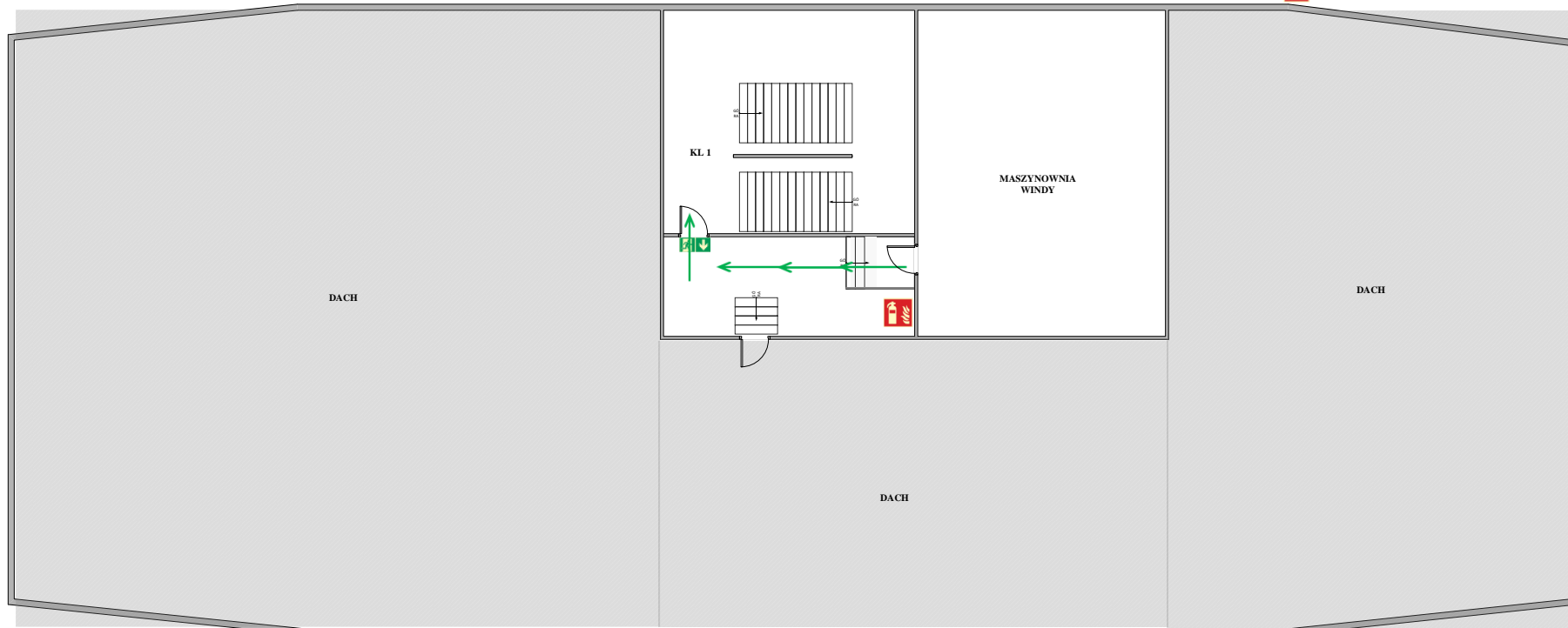
Rozmieszczenie urządzeń przeciwpożarowych oraz kierunków ewakuacji W BUDYNKU C-7 POLITECHNIKI WROCŁAWSKIEJ XI PIĘTRO CZ. A/B
