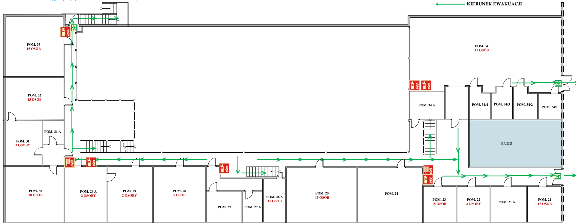
Rozmieszczenie urządzeń przeciwpożarowych oraz kierunków ewakuacji W BUDYNKU C-7 POLITECHNIKI WROCŁAWSKIEJ I PIĘTRO CZ. C
