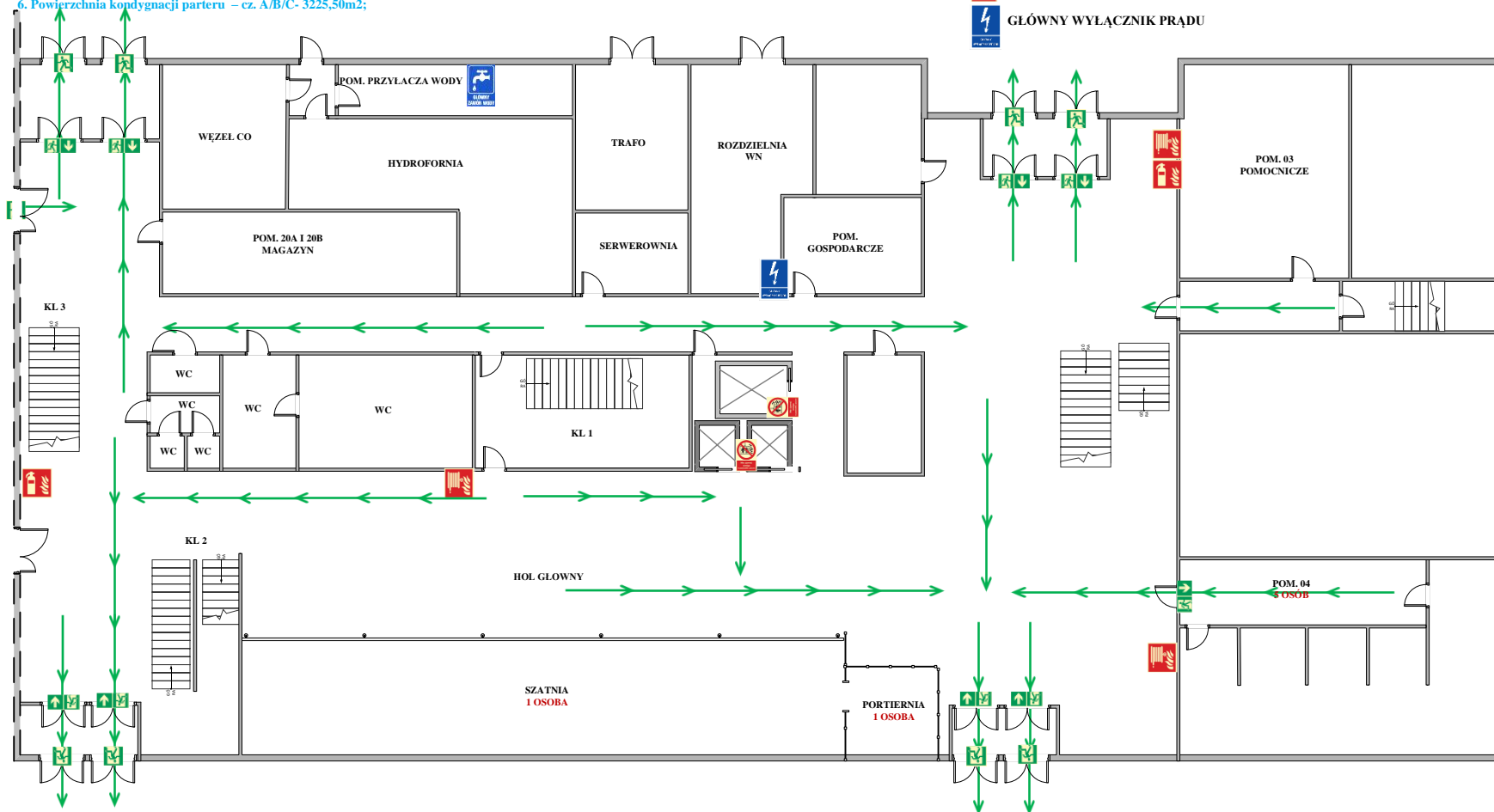
Rozmieszczenie urządzeń przeciwpożarowych oraz kierunków ewakuacji W BUDYNKU C-7 POLITECHNIKI WROCŁAWSKIEJ PARTER CZ. A/B
