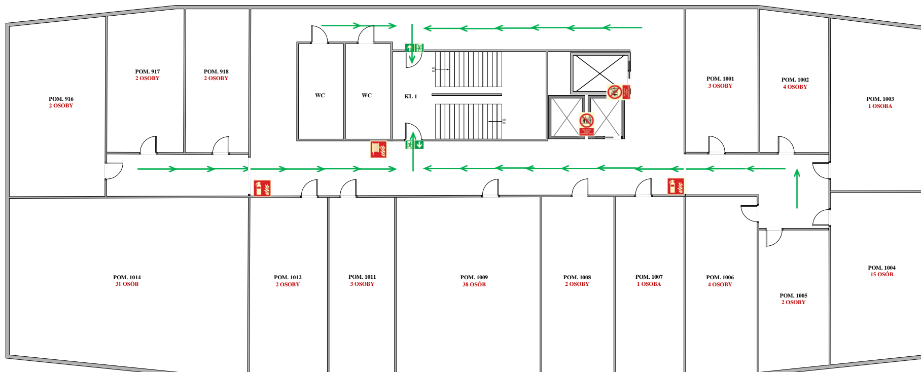
Rozmieszczenie urządzeń przeciwpożarowych oraz kierunków ewakuacji W BUDYNKU C-7 POLITECHNIKI WROCŁAWSKIEJ X PIĘTRO CZ. A/B
