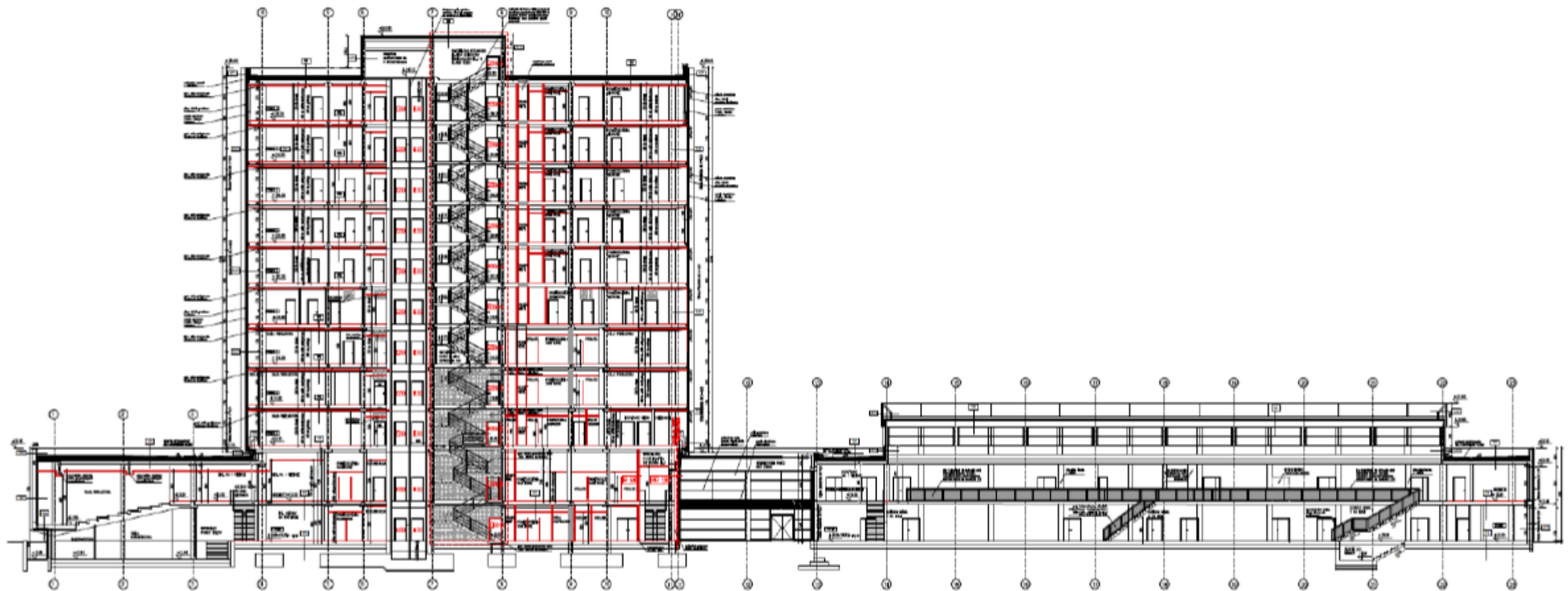
PRZEKRÓJ A-A BUDYNKU C-7 POLITECHNIKI WROCŁAWSKIEJ
