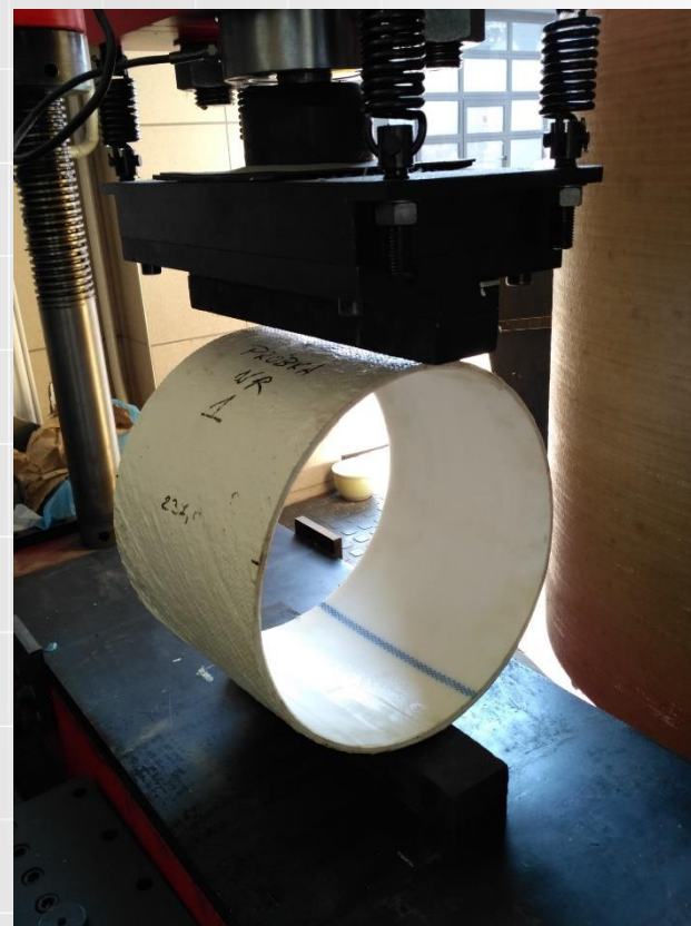
badanie wytrzymałościowe – sztywność obwodowa
