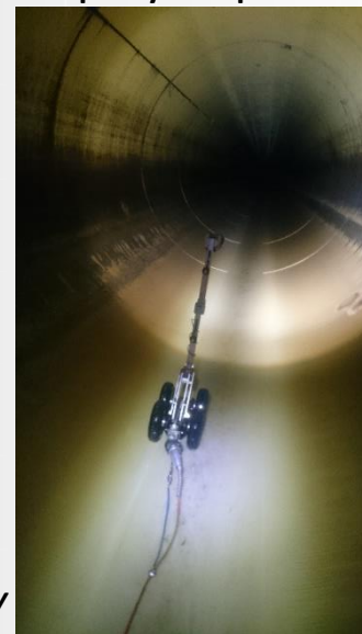
inspekcja CCTV
